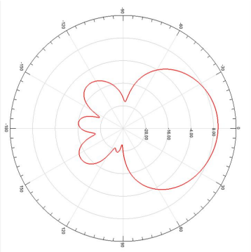
水平面波束宽度
