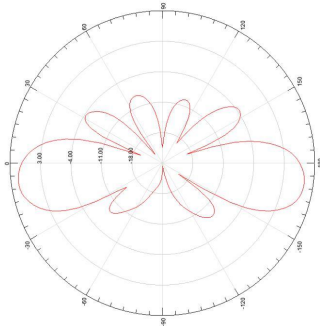
垂直面波束宽度
