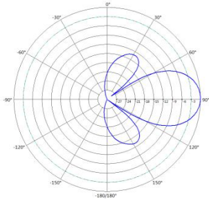
垂直面波束宽度
